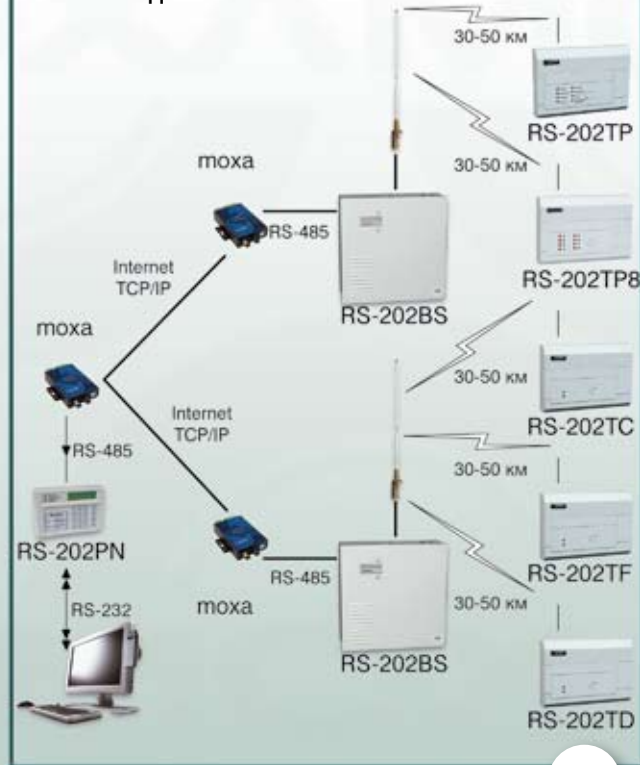
Схема соединений
